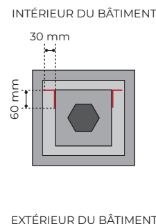
PLATINE DE PRÉ-SCÈLEMENT + POTEAU + CORNIÈRES EN L (VUE DE DESSUS)
