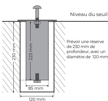
PLATINE DE PRÉ-SCÈLEMENT (VUE DE FACE)
