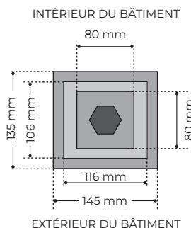
PLATINE DE PRÉ-SCÈLEMENT + POTEAU (VUE DE DESSUS)
